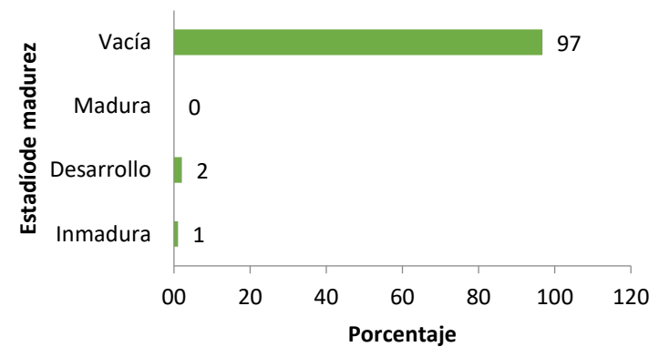
DESARROLLO GONADAL
