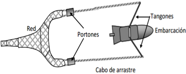
ARTE DE PESCA Red de arrastre “Changa”
